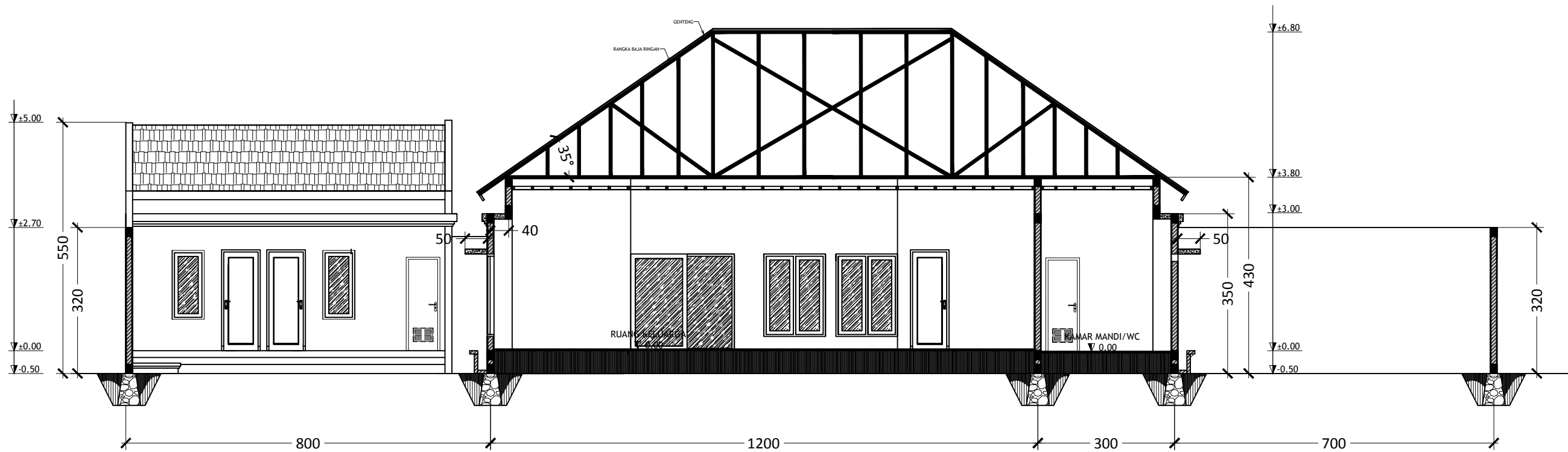
POTONGAN A SKALA 1:100
